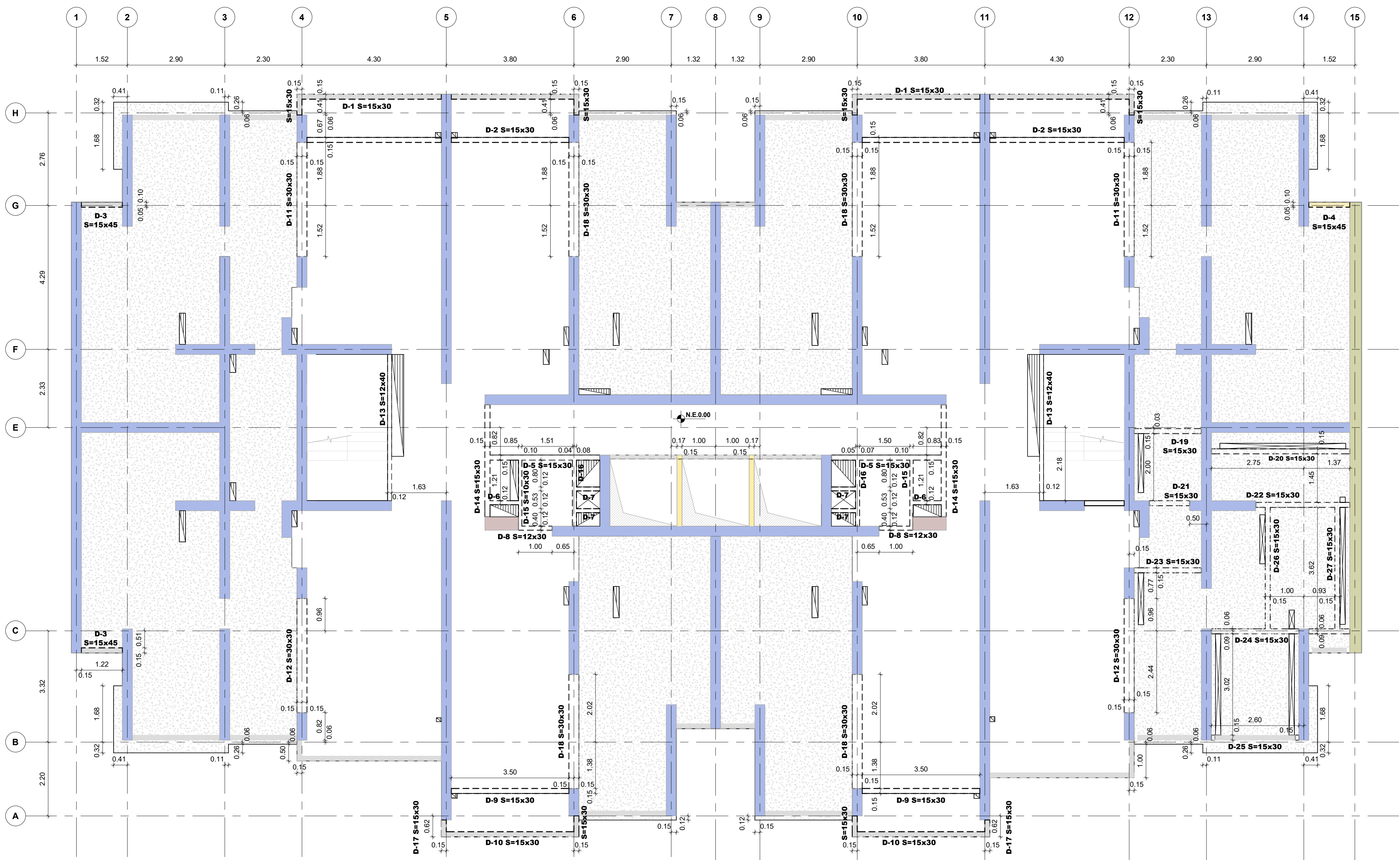
PLANTA LOCALIZACIÓN DE DINTELES PISO 1 Escala 1 : 75
